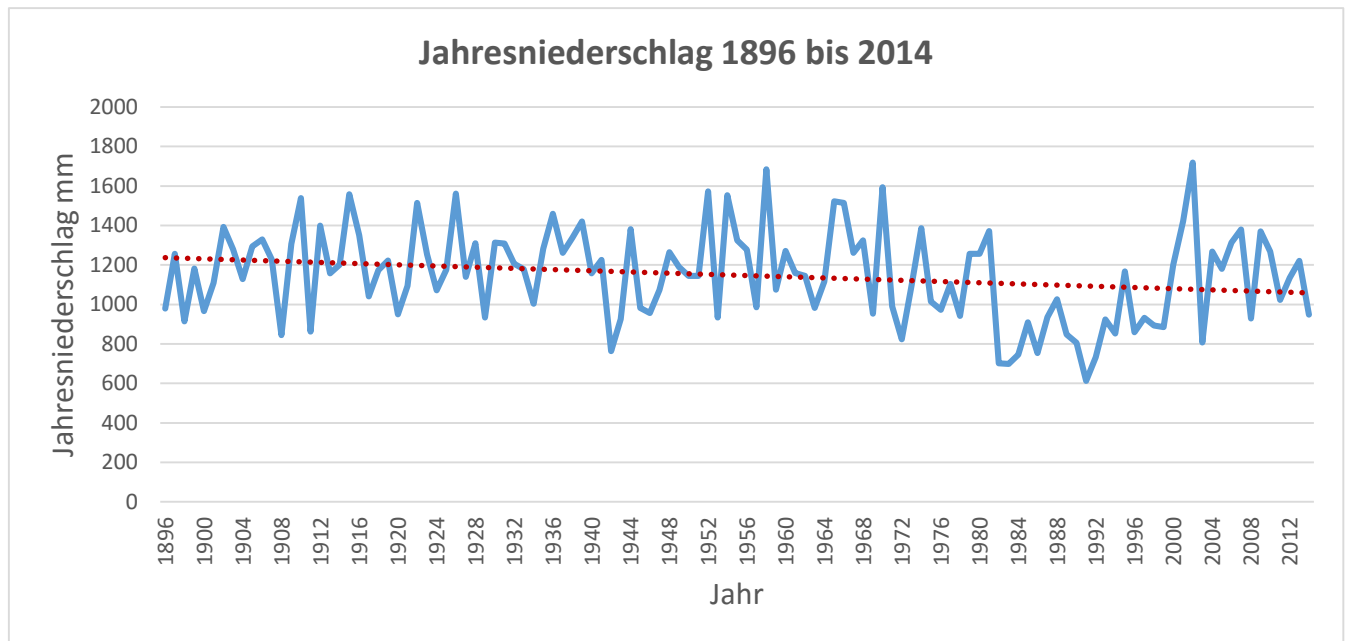
Abbildung 4: Entwicklung der Jahresniederschläge
