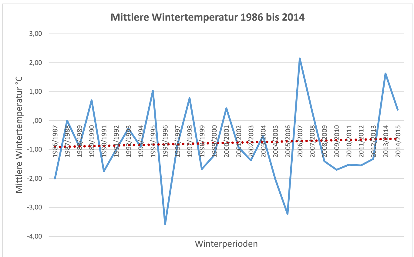
Abbildung 2: Entwicklung der mittleren Wintertemperatur
