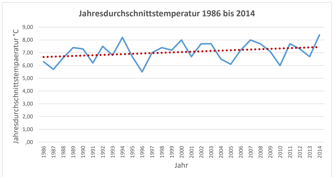
Abbildung 3: Entwicklung der Jahresdurchschnittstemperatur
